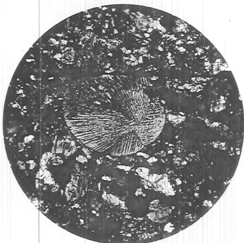
Fig. 3. — Chondre d'enstatite.
