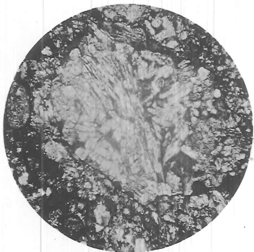
Fig. 1. — Agrégat d'olivine.
