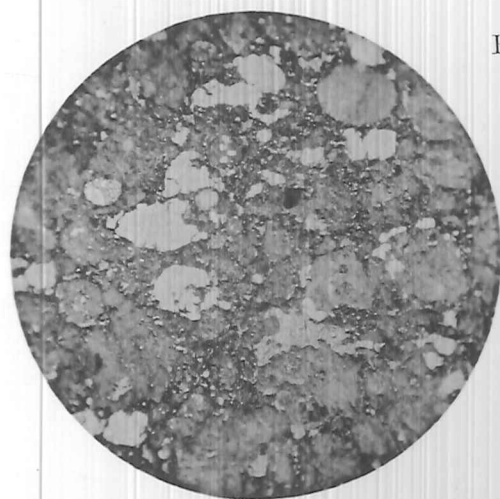
Fig. 6. — Plages métalliques.
