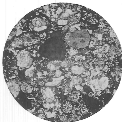
Fig. 2. — Pyroxènes rhombiques.
