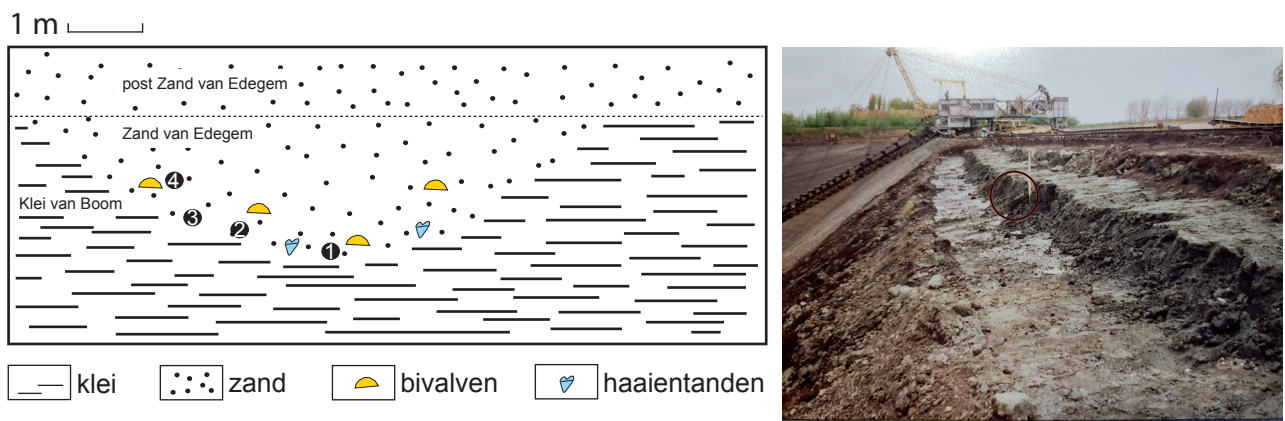
Figuur 6. Situering van de zandlens in de kleigroeve ARGEX te Kruibeke en profieltekening van het ontsloten Mioceen in 2007. De witte cijfers in zwarte cirkels verwijzen naar de genomen sedimentstalen, nu in KBIN. Het maatstreepje geldt voor zowel de lengte als de diepte van de geul.
