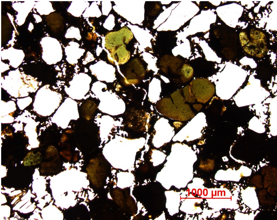
slijpplaatje, grote afgeronde witte vlekken, ca 500µm groot zijn kwartskorrels, kleinere en hoekige witte vlekken zijn grote poriën, groene
